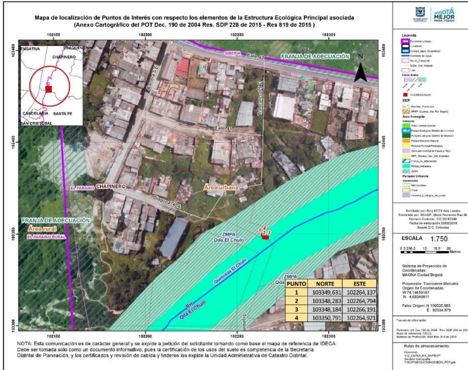
Imagen 1. Cartografía de las intervenciones proyectadas en el cauce de la quebrada El Chulo.
